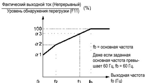
Характеристики охлаждения двигателя со встроенным самоохладяющим вентилятором
